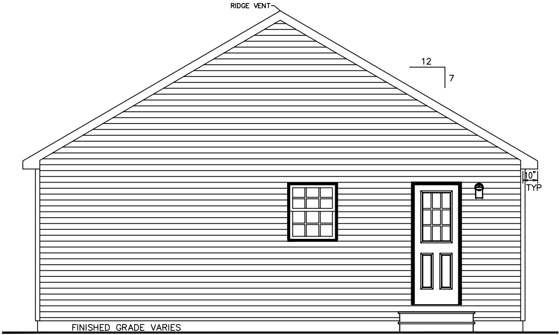
RIGHT ELEVATION
