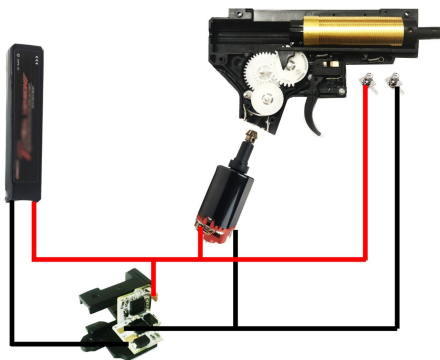
普通接线图
