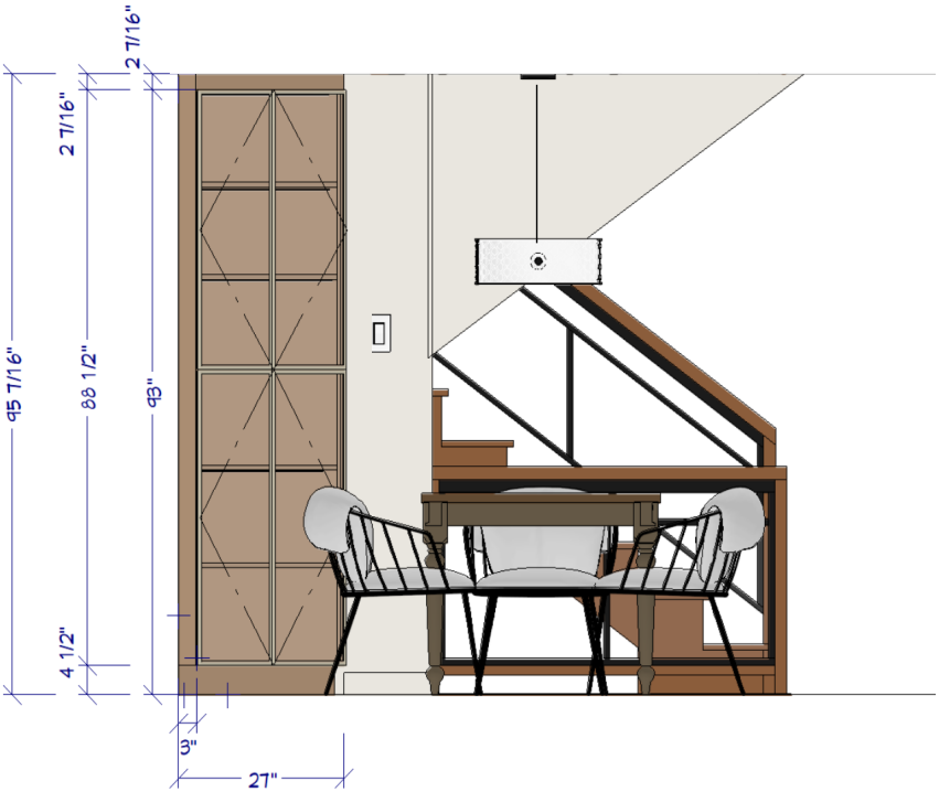
Elevation 7
