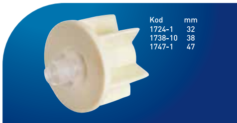
Kod mm 1724-1 32 1738-10 38 1747-1 47 Ürün Adı /Product name /Наименование продукта 32'lik Yaylı Boru Burcu Заглушка верхней трубки ( 32 мм ) End plug (32 mm)
