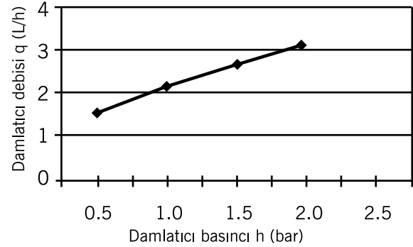
Ø17mm 2,2 debili damlama borularının basınç-debi ilişkisi
