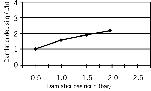
Ø17mm 1,6 debili damlama borularının basınç-debi ilişkisi
