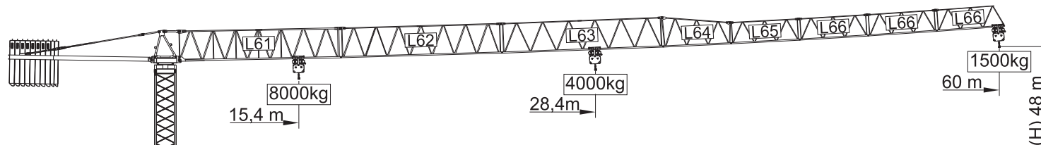
Yük Diagramı Cargas.Loads.Lasten.Charges.Cargas.Carichi.Yükler. ГРУЗОПОДЪЕМНОСТЬ
