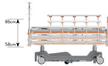
58-86 cm Yükseklik Hareketi 58-86 cm Height Movement
