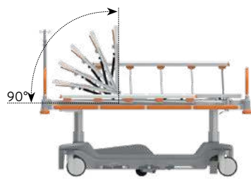
90° Sırt Hareketi 90° Backrest Movement
