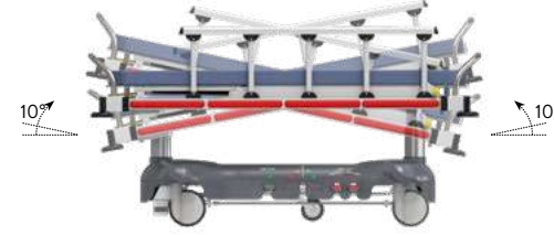
10° Trendelenburg / Ters Trendelenburg 10° Trendelenburg/Antitrendelenburg
