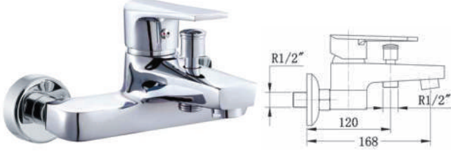
Banyo Bataryası
