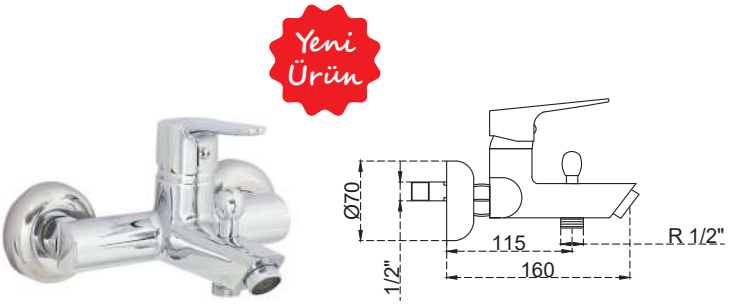
Banyo Bataryası 29.01.100
