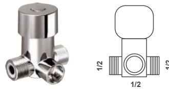
Mixer Ayırıcı 01.02.400
