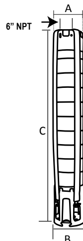
Acoplamiento NEMA 8"
