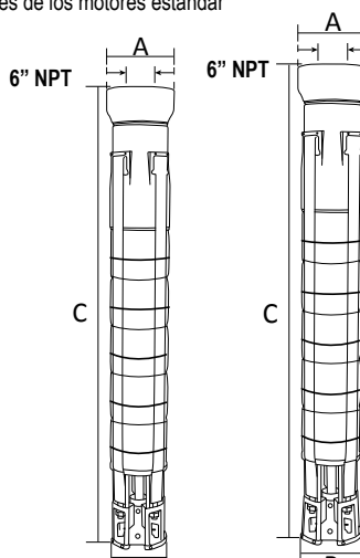
Acoplamiento NEMA 6"
