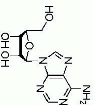
Adenosine
