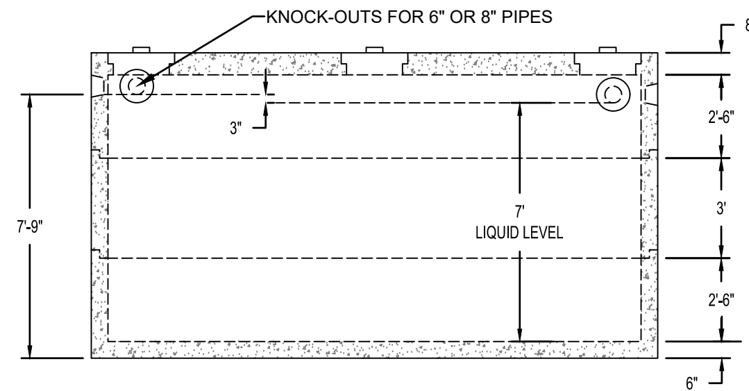
7, 500 GALLON ANOXIC TANK
