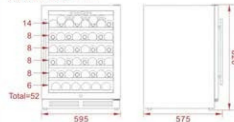
SRW-54S Product(W*D*H)mm
