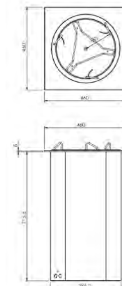
Modelo 65 platos
