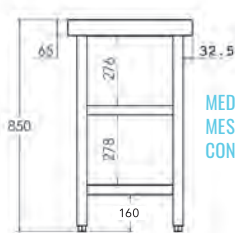
MEDIDAS MESA CENTRAL CON ESTANTE
