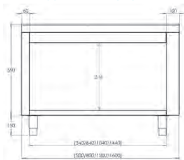
MEDIDAS SELF INFANTIL NEUTRO
