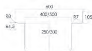
MEDIDAS CUBETA
