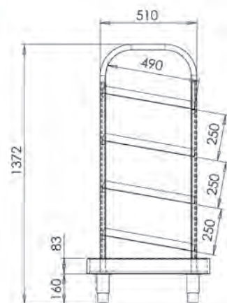
MEDIDAS DISPENSADOR
