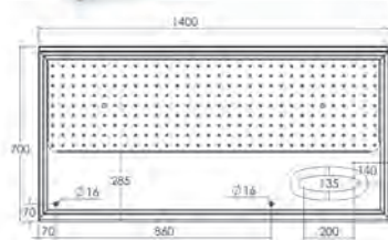
MEDIDAS MESA PREPARACIÓN DE CARNE Y PESCADO
