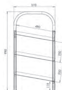
MEDIDAS DISPENSADOR
