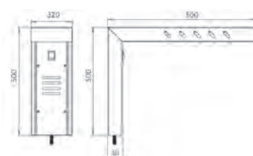
MEDIDAS PANTALLA DE CALOR
