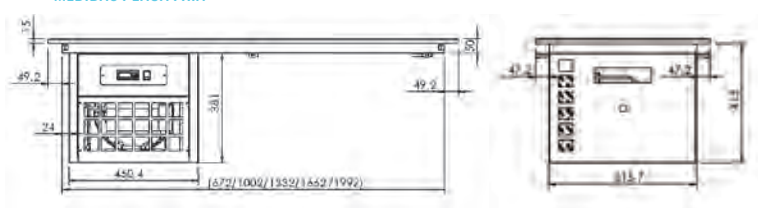
MEDIDAS PLACA FRÍA
