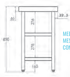
MEDIDAS MESA CENTRAL CON ESTANTE
