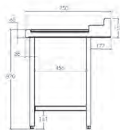
MEDIDAS MESA MURAL
