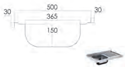
MEDIDAS CUBETA
