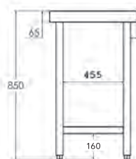
MEDIDAS MESA CENTRAL CON ESTANTE
