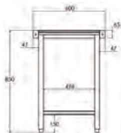
MEDIDAS MESA CENTRAL
