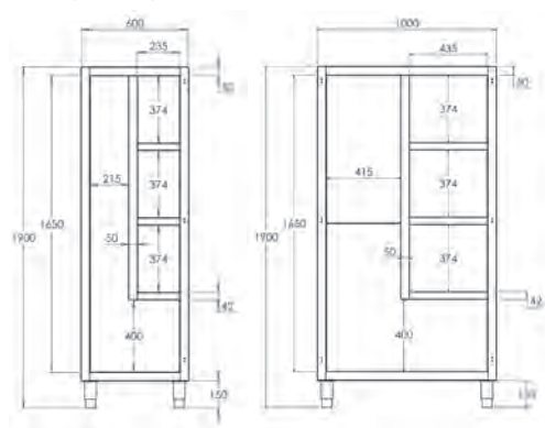
MEDIDAS ARMARIO DE PIE
