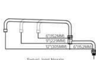
Swivel-Joint Nozzle
