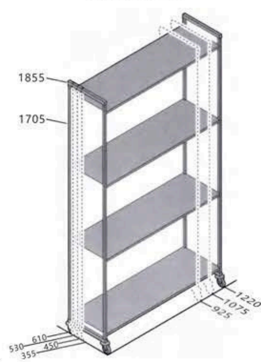
移动式架体尺寸 Mobile Unit Size
