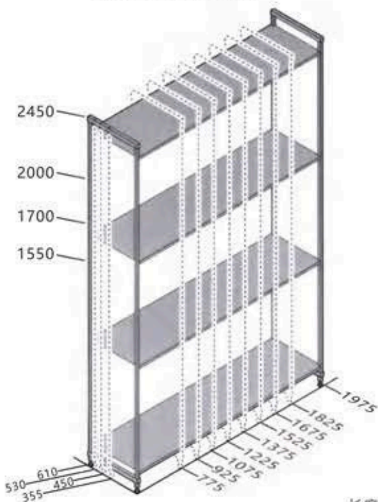
固定式架体尺寸 Stationary Unit Size
