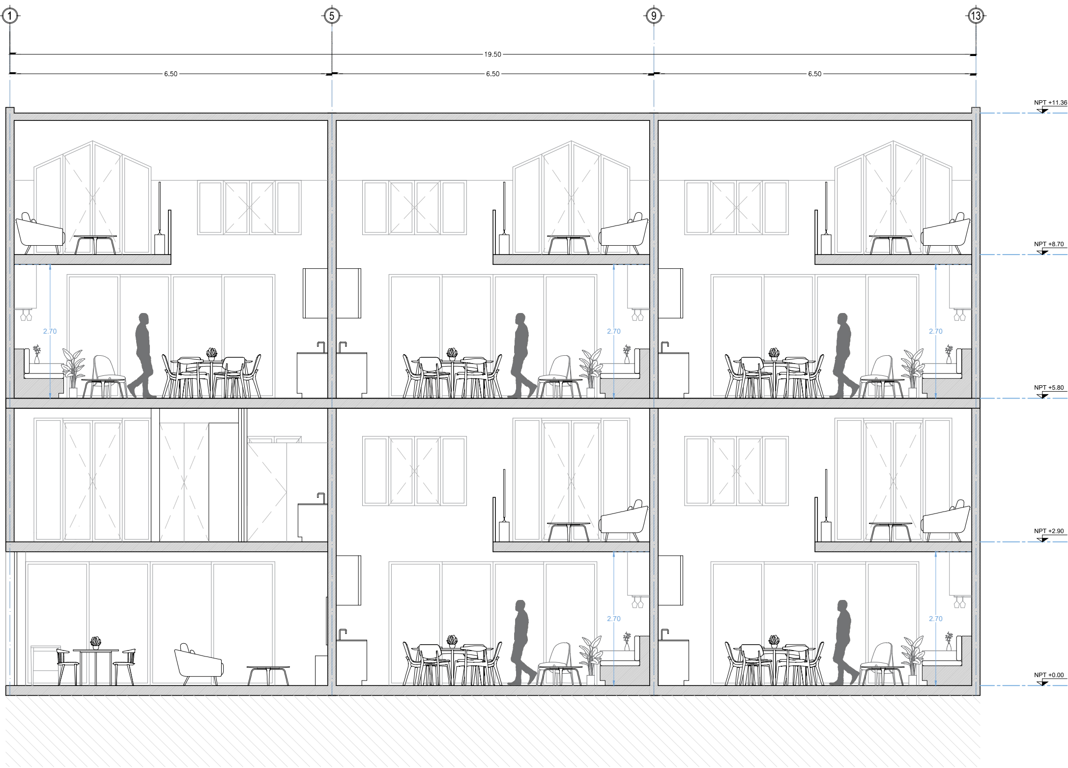
Corte A-A'
