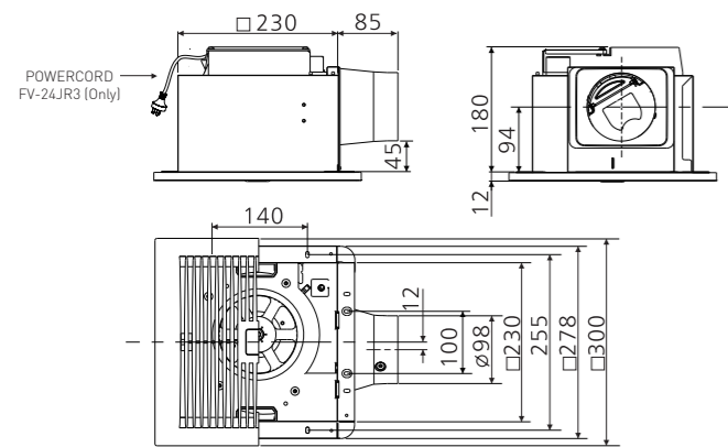
FV-24JR3 & FV-24JA3
