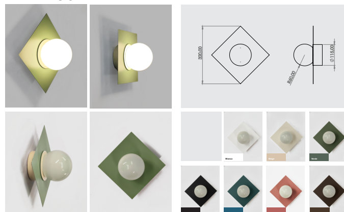
APLIQUE DE PARED AP W30
