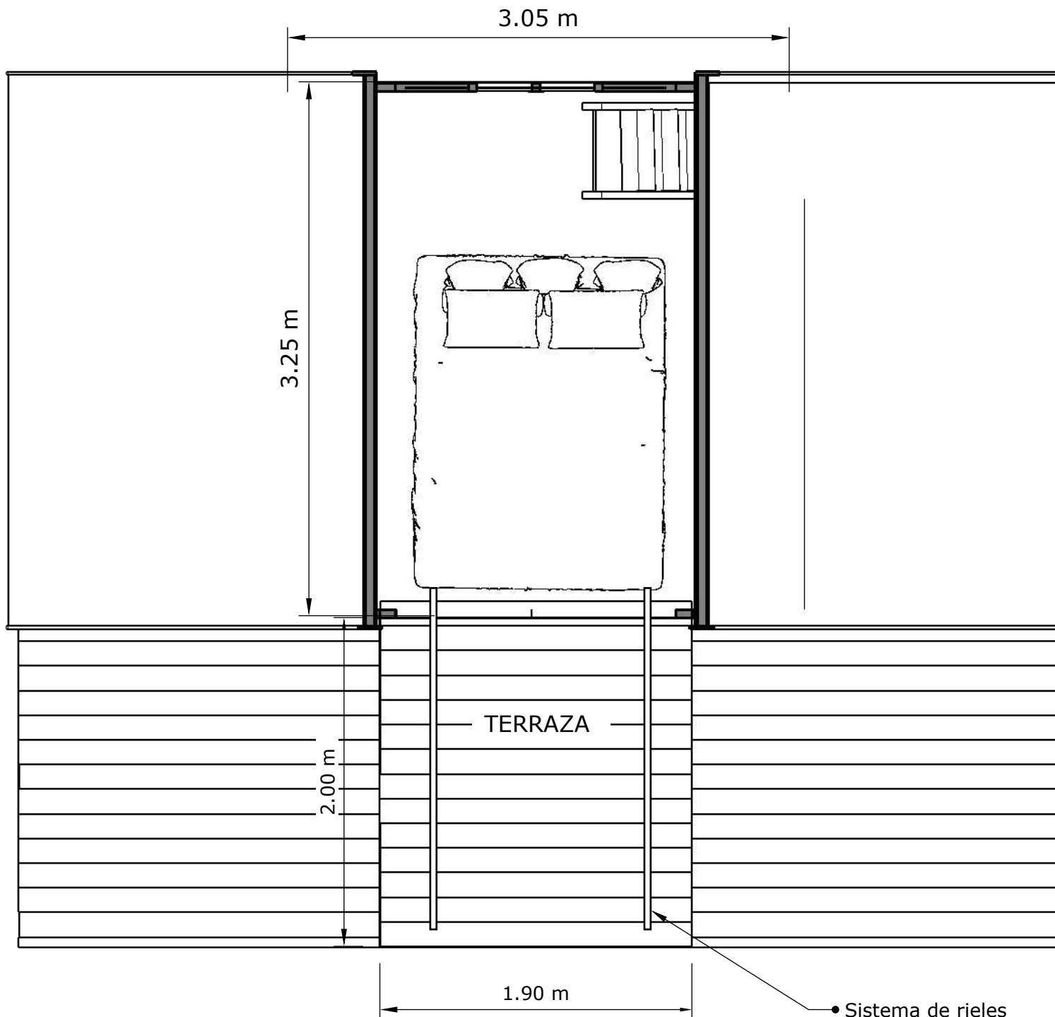
Distribución Planta Alta
