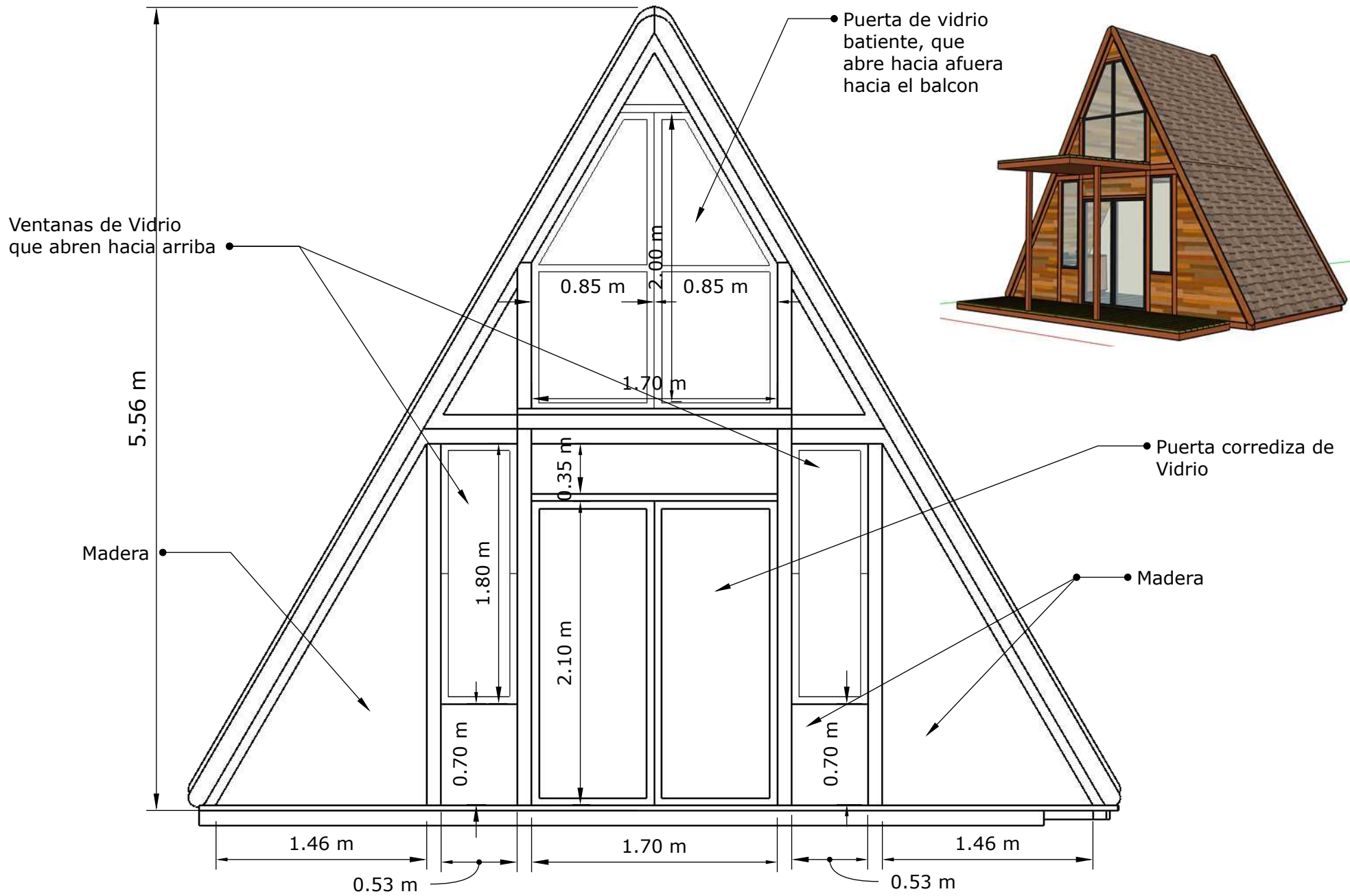
Fachada Frontal
