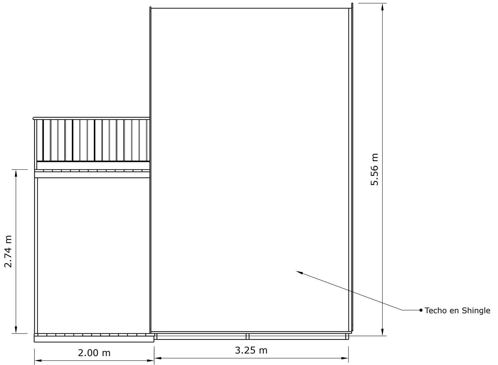
Fachada Lateral
