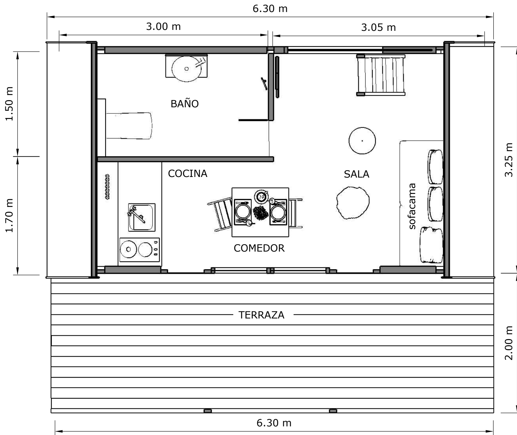
Distribución Planta Baja
