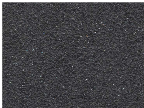
4203 | Biotite
