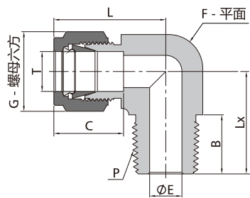
卡套阳螺纹弯头
