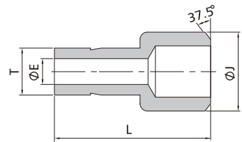
卡套管+焊接转换接头
