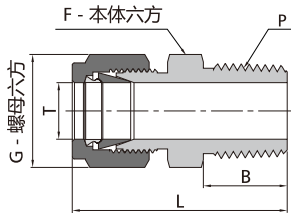
卡套阳螺纹穿孔接头
