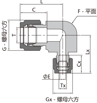
卡套变径弯头
