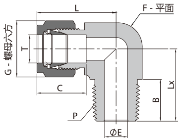
卡套阳螺纹弯头
