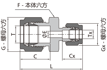
卡套直通变径接头
