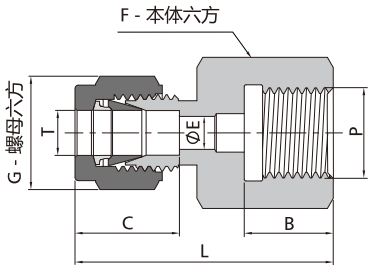
转换至日本压力表螺栓
