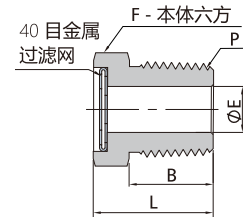
40目300系列不锈钢过滤网组件
