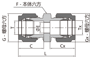
卡套直通转换接头
