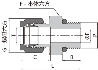
卡套阳螺纹接头
