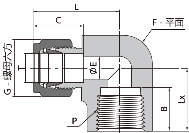
卡套阴螺纹接头
