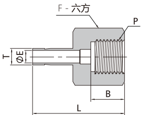
卡套管+阴螺纹转换接头
