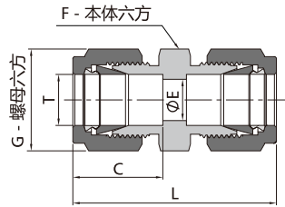
卡套直通接头
