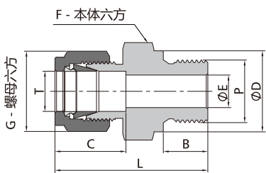
卡套阳螺纹接头
