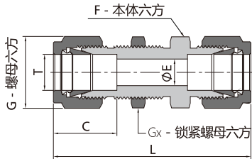
卡套直通穿板接头
