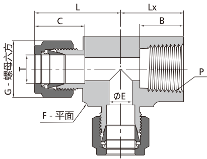
主管阴螺纹卡套三通
