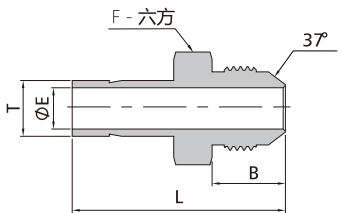
卡套管+阳螺纹转换接头
