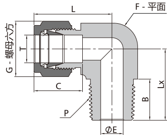
卡套阳螺纹弯头
