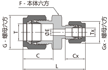
卡套直通变径接头
