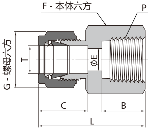
卡套阴螺纹接头
