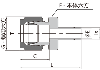
卡套+卡套管转换接头
