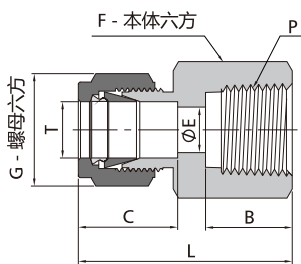
卡套阴螺纹接头
