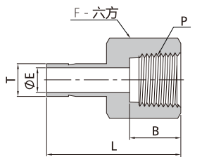
卡套管+阴螺纹转换接头
