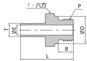
卡套管+阳螺纹转换接头
