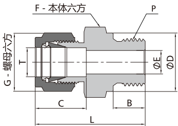
卡套阳螺纹接头
