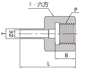
转接至日本压力表螺栓
