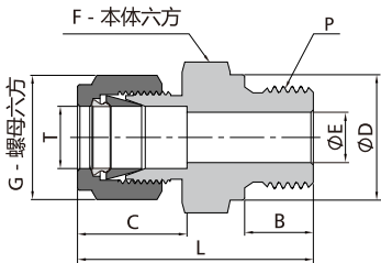
英制I Tube 管
