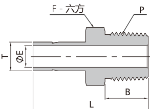
卡套管+螺纹阳转换接头
