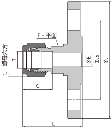
法兰转换接头
