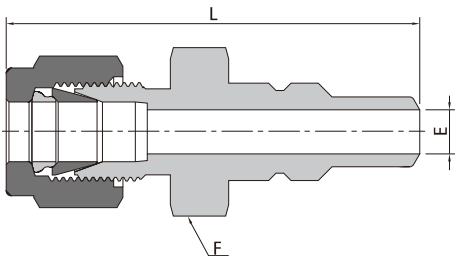
卡套
