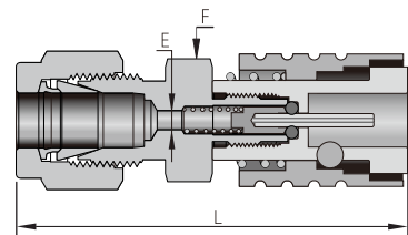
卡套
