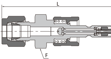
卡套
