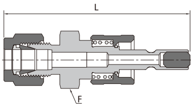
卡套
