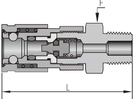
NPT外螺纹
