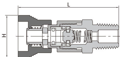
NPT阳螺纹
