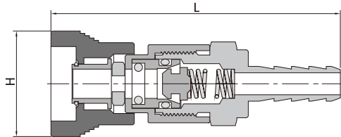
软管端口
