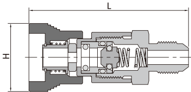
37°扩口阳螺纹
