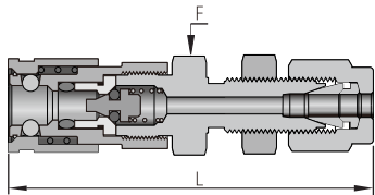
卡套
