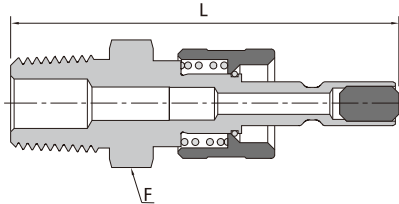
BSPT 阳螺纹
