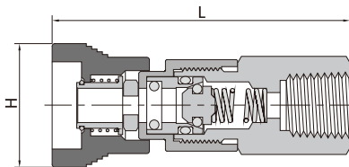
NPT阴螺纹
