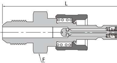
37°扩口阳螺纹
