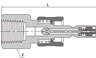
BSPT阴螺纹
