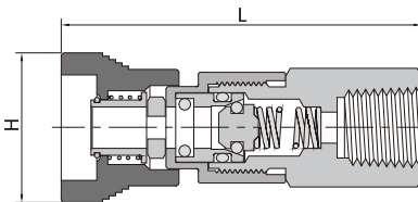
BSPT阴螺纹
