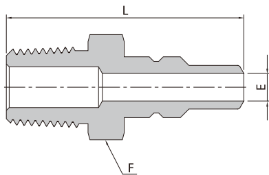
BSPT 阳螺纹
