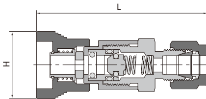
卡套端口
