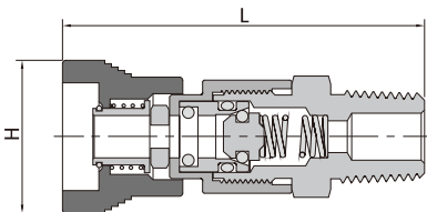
BSPT阴螺纹
