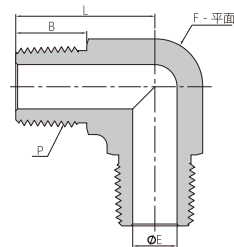
阳螺纹弯通接头
