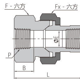
阴螺纹活接头
