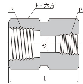
六方阴螺纹接头
