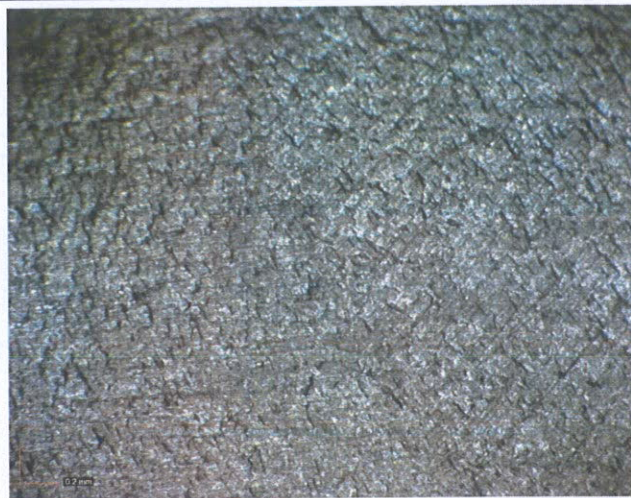
177475-2-2 金相图/Metallograph 20X
