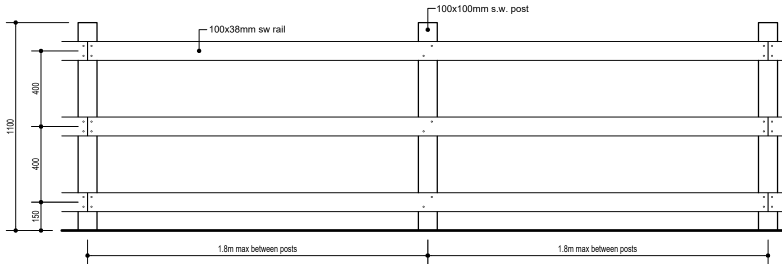
ELEVATION
