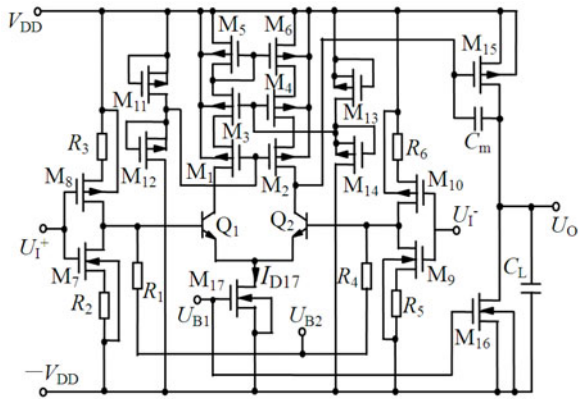
(b) A 3 : BiCMOS op amp
