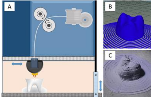
Şekil 5. Kaynaşmış Biriktirme Modelleme (FDM). (A) FDM Yazıcı. (B) Diş Kronu CAD Dosyası. (C) Diş Kronu FDM (Khorsandi ve ark., 2021).
