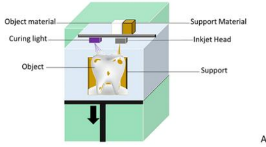
Şekil 4. (A) Fotopolimer püskürtme (Khorsandi ve ark., 2021).
