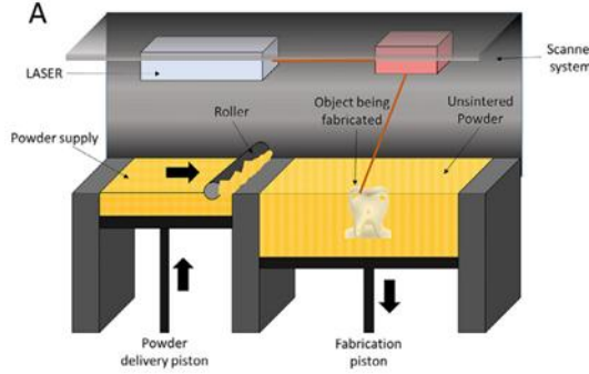
Şekil 3. Seçici lazer sinterleme (SLS). (A) SLS ile Hareketli Parsiyel Protez İskeletinin Tasarımı ve Üretimine İlişkin Çizimler (Khorsandi ve ark., 2021).
