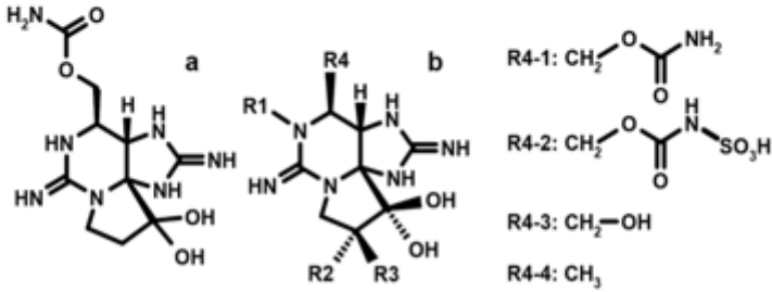
Şekil 2. (a) Saksitoksin yapısı; (b) saksitoksinin ve gonyautoksinin genel yapısı
