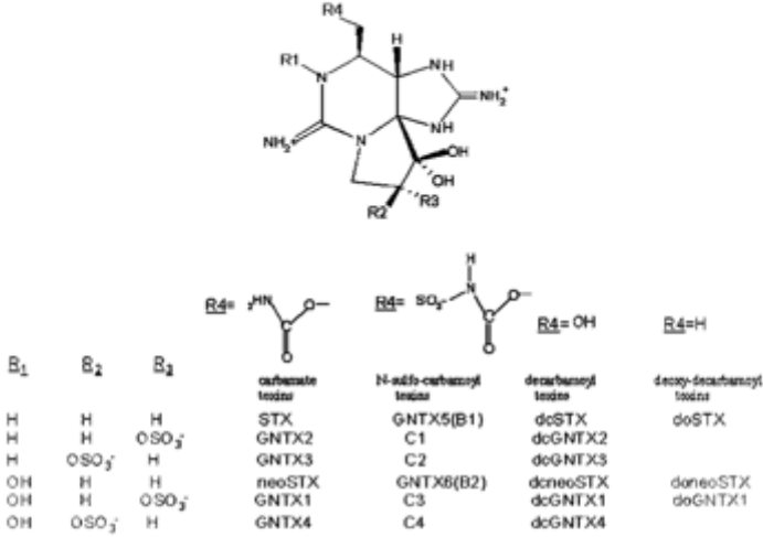
Şekil 1. Saksitoksin ve Saksitoksin grupları (Mons vd., 1998; Quilliam vd., 2001)
