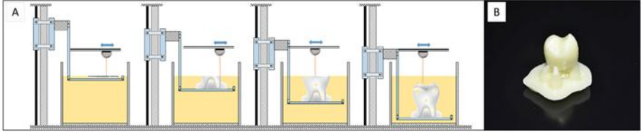
Şekil 1. SLA. (A) Katman Katman Baskı İşlemi. (B) Destekler Çıkarılmadan ve Cilalanmadan Önce Stereolitografi ile Basılmış Bir Kron Örneği (Khorsandi ve ark., 2021).
