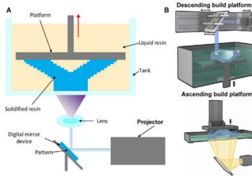
Şekil 2. DLP. (A) Yazıcı Bileşenlerinin ve Baskı Prosedürünün Şeması. (B) DLP Yönteminde İki Tür Platform Hareketinin Gösterilmesi (Khorsandi ve ark., 2021).
