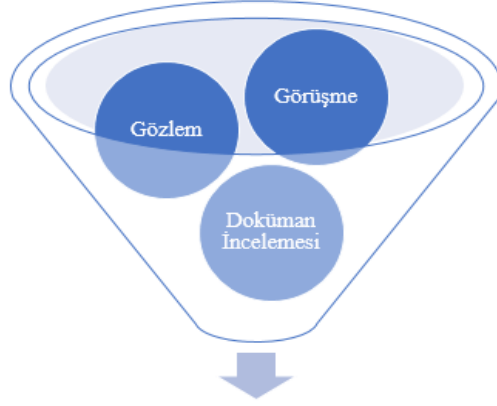
Şekil 4.1. Veri Üçgenlemesi
