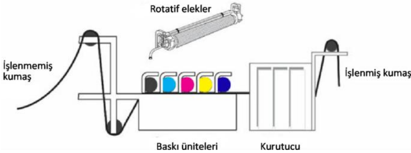
Şekil 11. Tekstil yüzeylerinde esansiyel yağ kapsülleme yüzeylerinin serigrafi baskı kullanılarak uygulanması
