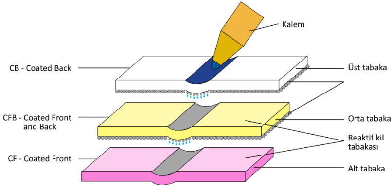
Şekil 3. Mikrokapsüllerin karbonsuz kopya kâğıdında kullanımı
