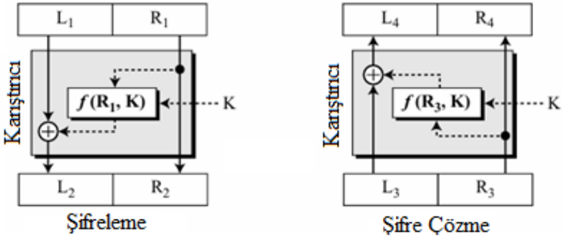
Şekil 2 Feistel tasarımının geliştirilmiş hali
