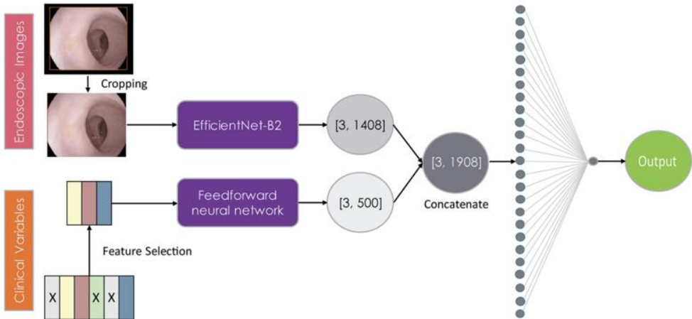
Şekil 7: Haak ve diğerlerinin birleşik model mimarisi (Haak ve ark., 2022a)
