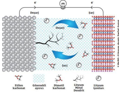
Şekil 12. Lityum metal pil yapısı [2]
