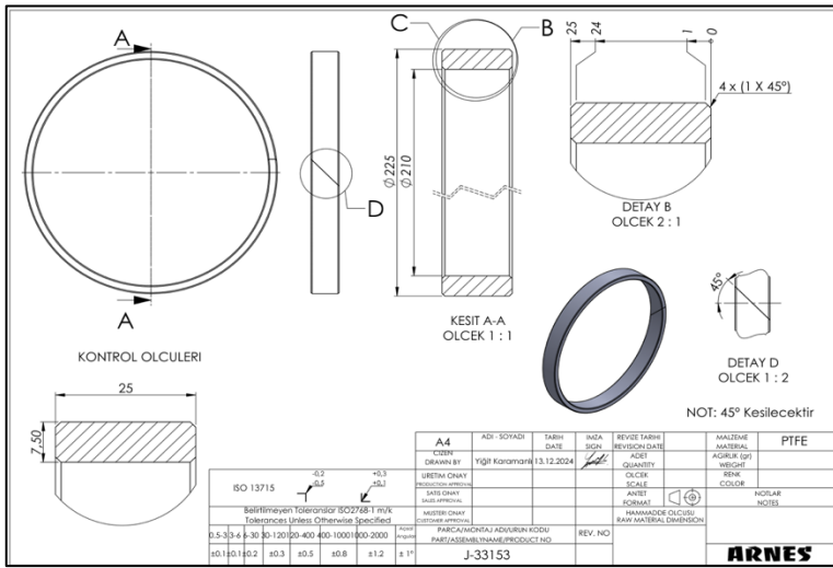
Şekil 1. Yataklama elemanı prototipinin teknik resmi
