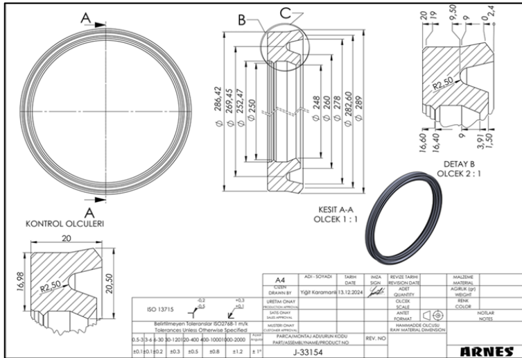
Şekil 2. Boğaz keçesi prototipinin teknik resmi
