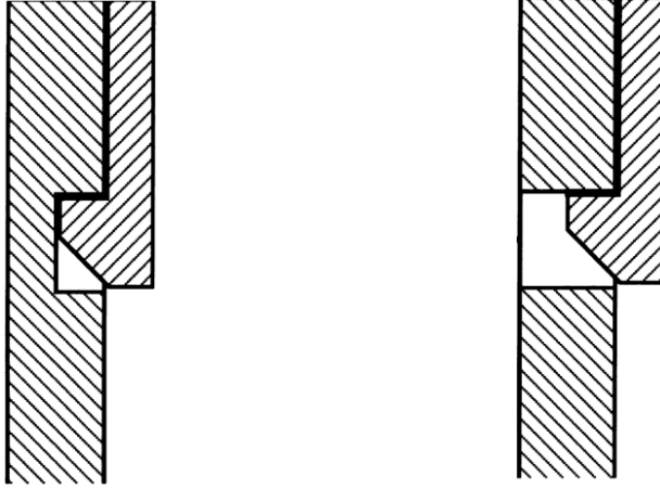
Şekil 3. Tahribatsız söküm prensibi: Elastik şekil bağı (form-fit) kullanılarak parçaların ve bağlantı elemanlarının zarar görmeden ayrıştırılması (Bode, 1996).
