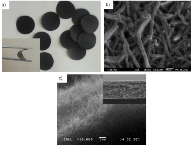
Şekil 3. (a) Esnek, serbest duran MWCNT buckypaper'lar, (b) buckypaper'ın yüzeyinden alınan FE-SEM görüntüsü ve (c) kesit bölgesinden alınan FE-SEM görüntüsü(Alaf et al., 2013a).
