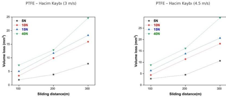
Şekil 7. 3 m/s ve 4.5 m/s hızda uygulanan aşınma testine ait hacimsel kayıplar
