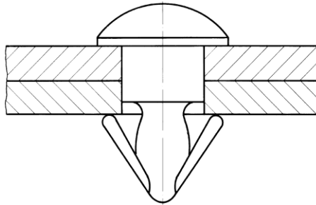
Şekil 8. Plastik parçalarda konsol tipi geçme bağlantı (snap-fit) mekanizmasının kesit görünüşü ve kilitleme (undercut) prensibi (Bode, 1996).
