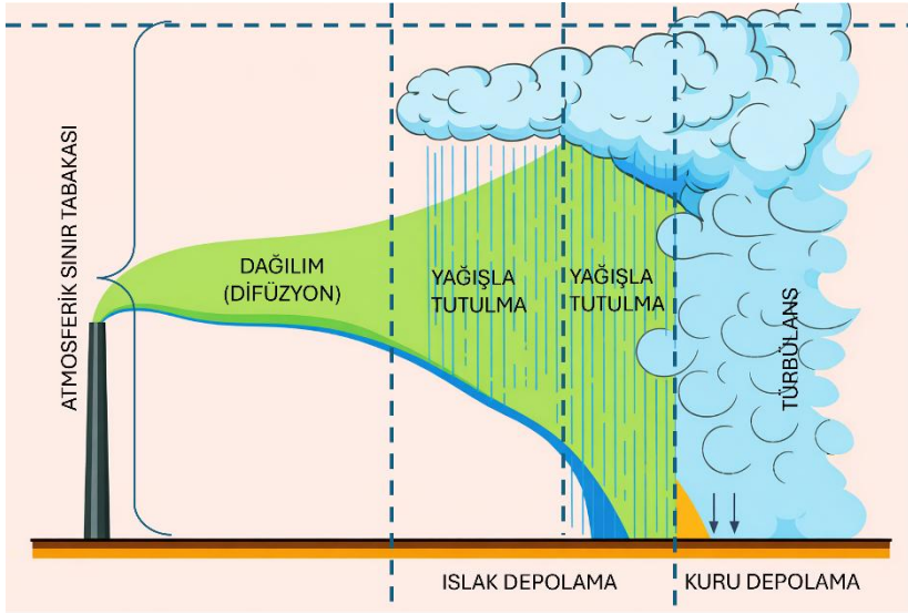
Şekil 15: Atmosferde yayılan kirleticilerin azalma mekanizmaları (Till ve Meyer, 1983).
