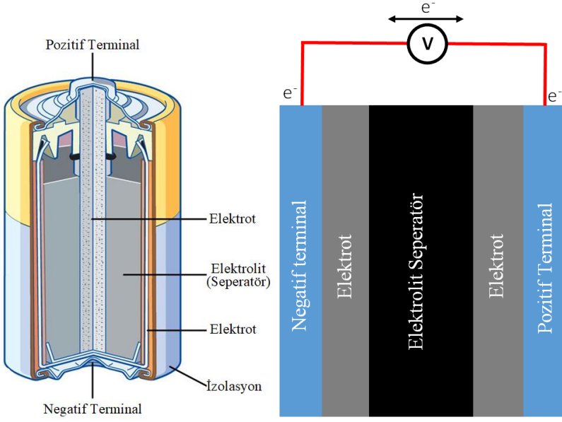
Şekil 9. Bataryaların genel yapısı
