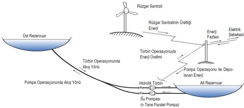
Şekil 1. Yüksek koda su pompalayarak enerji depolama yönteminin çalışma yapısı (Ünver, 2015)
