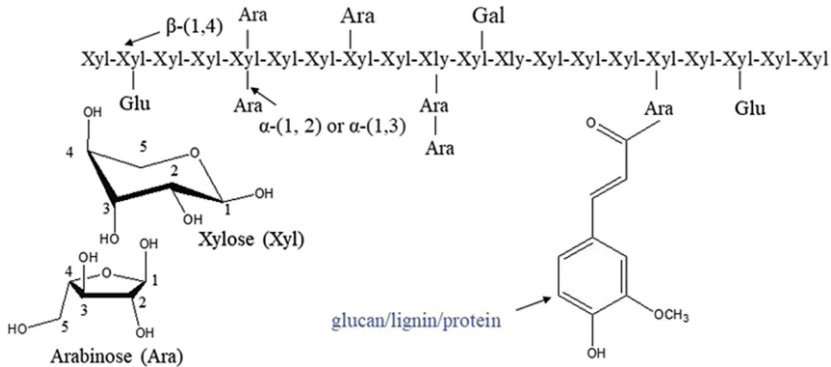
Şekil 1. Arabinoksilanların genel yapısı (Adams vd., 2004).
