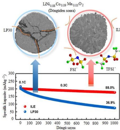
Şekil 13. Lityum metal pilin kapasite durumu [2]
