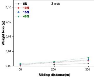
Şekil 6. 3 m/s ve 4.5 m/s hızda uygulanan aşınma testine ait kütleli kayıplar
