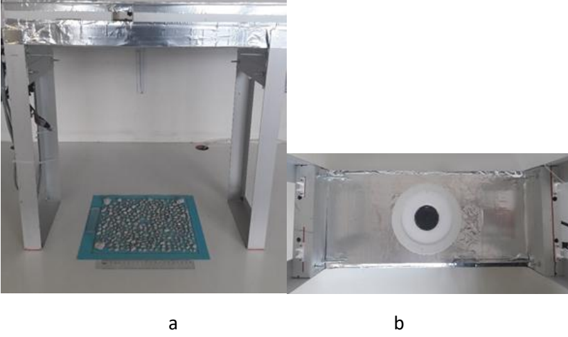
Şekil 1 Görüntü alma düzeneği a) Önden görünümü ve koyu arka fon üzerindeki kırmataş agrega numunelerinin yerleşimi, b) Alttan görünümü, siyah renkli merkezdeki objektif ve objektifi saran beyaz renkli led aydınlatmanın yerleşimi
