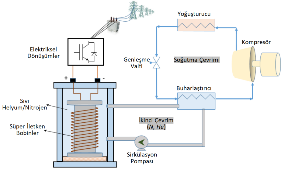
Şekil 12. Süperiletken manyetik enerji depolama sisteminin çalışma yapısı (Nikolaidis & Poullikkas, 2017)
