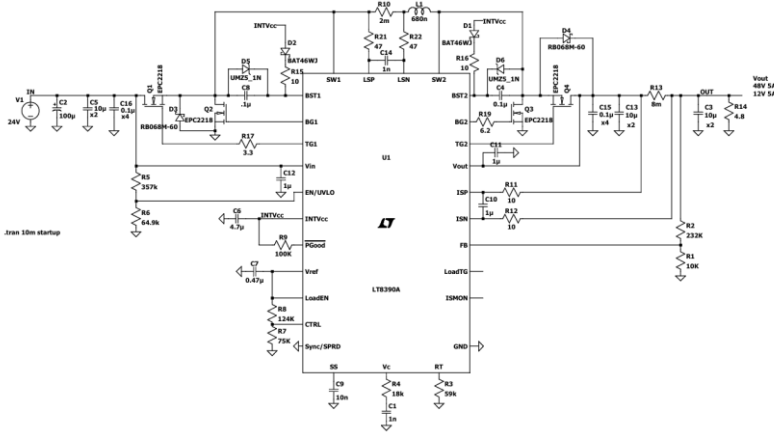
Şekil 2. LT8390A tabanlı senkron buck–boost dönüştürücünün LTSpice devre modeli
