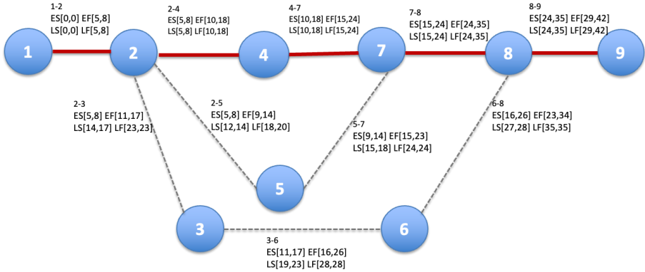
Şekil 1: Gri CPM modeli ağ diyagramı (AoA)
