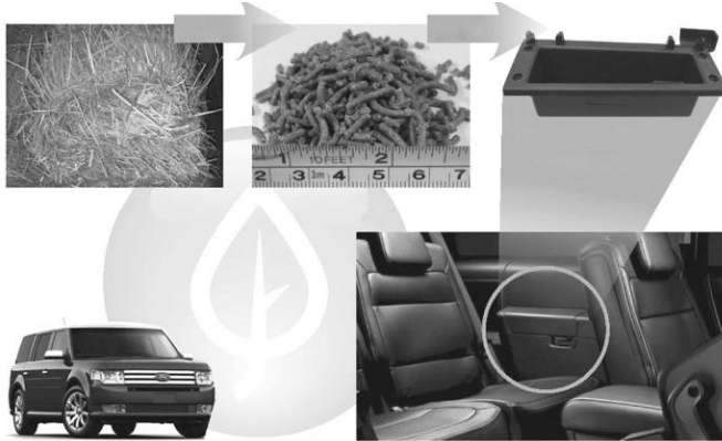
řekil 5. Ford esnek amurluk kaplama paneli, saklama blmesi ve kapak hattı tertibatında doğıal elyaf kullanımına dair bir rnek (%20 buğday samanı takviyeli PP). (Akampumuza, Wambua, Ahmed, Li, Qin, 2016)
