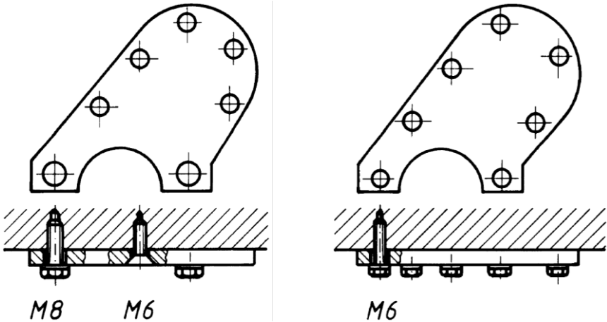
Şekil 2. Montaj verimliliğini artırmak için bağlantı elemanlarında standardizasyon: Farklı vida başları (sol) yerine tek tip bağlantı elemanı kullanımı (sağ) (Bode, 1996).
