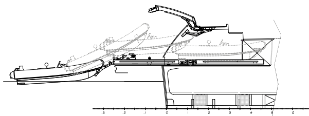
SEZIONE GARAGE
