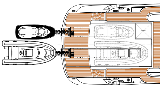
PIANTA GARAGE
