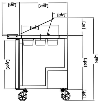
SIDE VIEW(1,2,3 DOOR)
