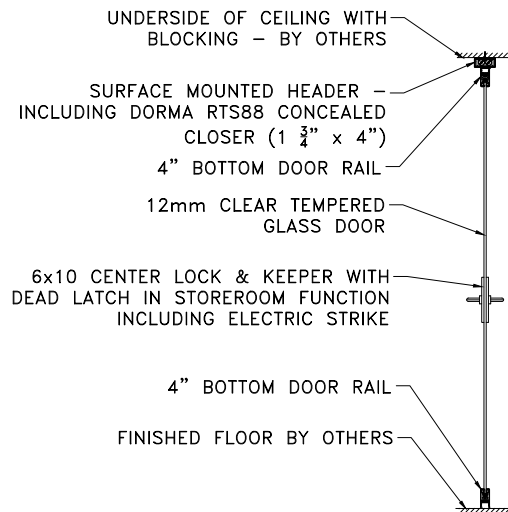
TYP. ENTRY DOOR & FRAME SECTION
