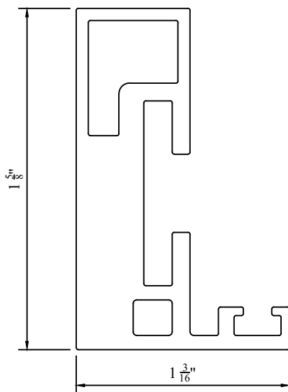
SLIMLINE DOOR PROFILE SECTION
