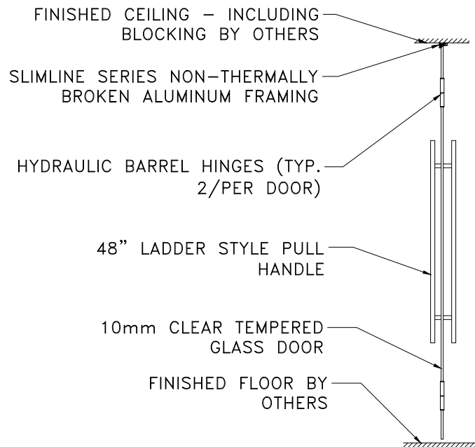
SLIMLINE DOOR & FRAME SECTION
