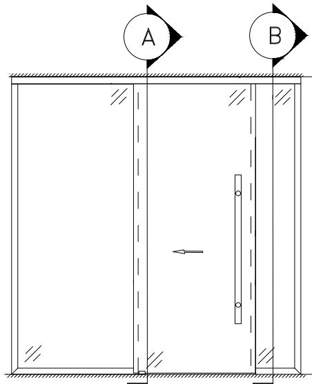
ELEVATION
