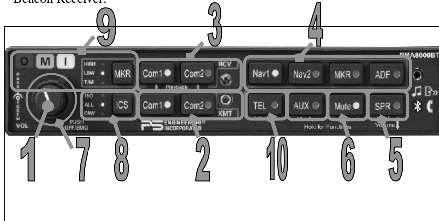
PMA8000BT controls
