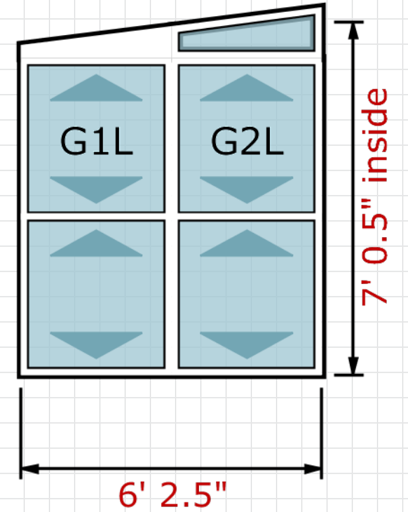
LEFT END - WIDTH
