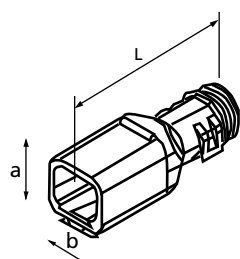
Receptacle 180°
