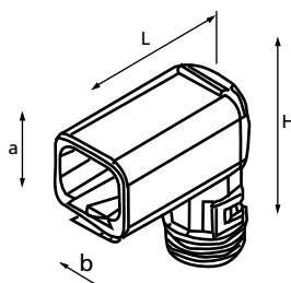
Receptacle 90°
