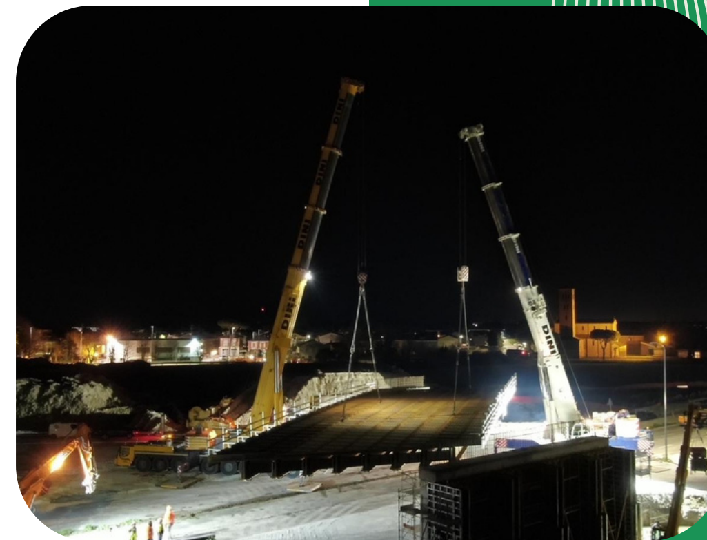
Opere realizzate nell'ambito dei lavori di ammodernamento della SS67 a Ravenna
