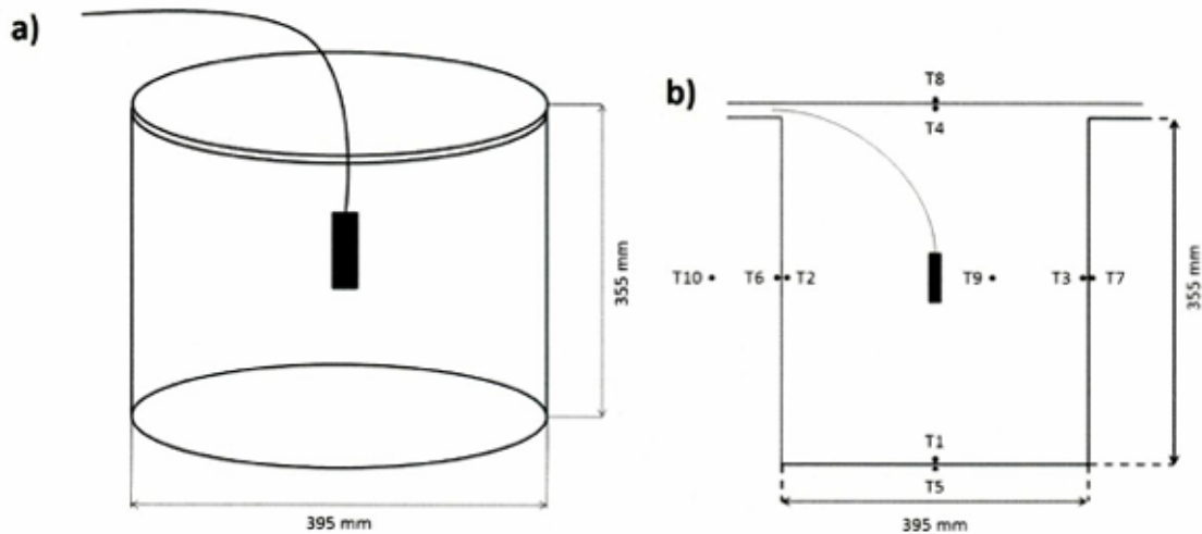
Şekil 1. Şematik görünüm a) 3D görünüm; b) termočiffler T_1, T_2, T_3 and T_4 iç yüzey sıcaklıkları; T_5, T_6, T_7 ve T_8 dış yüzey sıcaklıkları, T_9 iç sıcaklık ve T_{10} dış sıcaklık
