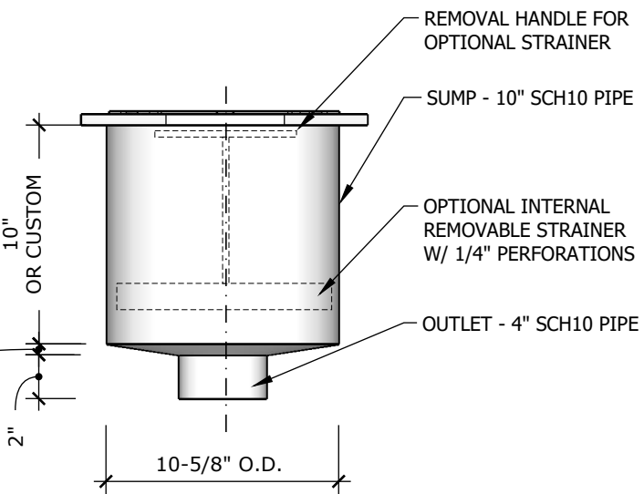
2 SUMP SIDE VIEW Scale: 1 1/2" = 1'-0"
