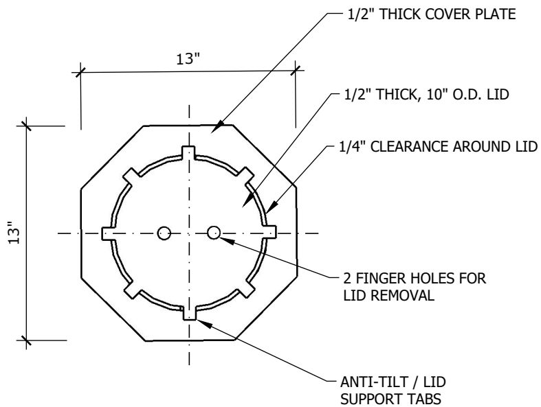
1 SUMP TOP VIEW Scale: 1 1/2" = 1'-0"
