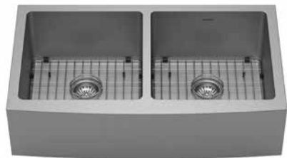
EL-88-PK1 36" x 22 1 / 4 " x 10"
