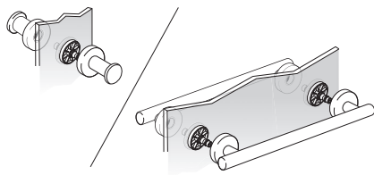
GLASS SHOWER ENCLOSURE HOLDER FOR HOOK / HOOK SOPORTE MAMPARA PARA COLGADOR / COLGADOR GLASS 6/8MM / VIDRIO 6/8MM
