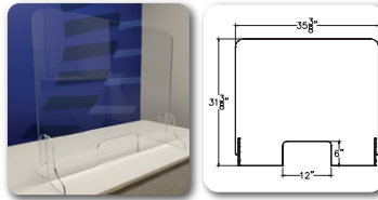
Sneeze Guard-A-36x32: (Part#: CI-SG-A-3x2.5)
