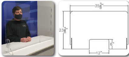
Sneeze Guard-A-36x24: (Part#: CI-SG-A-3x2)
