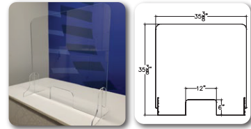
Sneeze Guard-A-36x36: (Part#: CI-SG-A-3x3)
