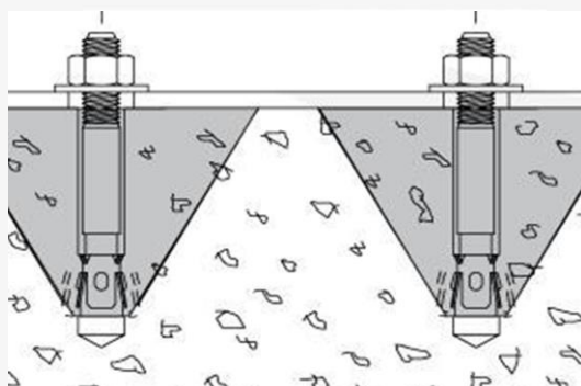
ANCLAJE AL SUELO POR EL INTERIOR DE LA CAJA
