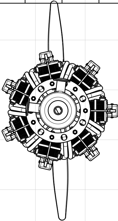
Left view Scale: 1:1
