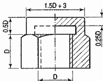
Cap nut FIG. 24-8
