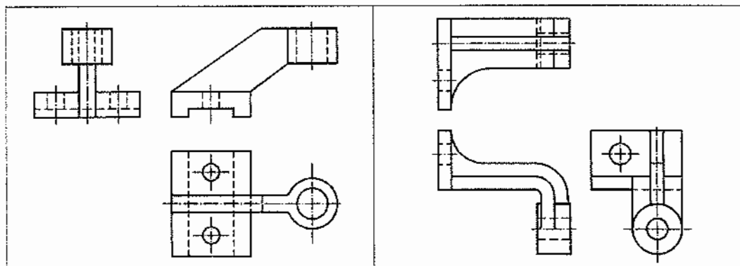
(Ex. 29. FIG. 20-61) FIG. 20-99
