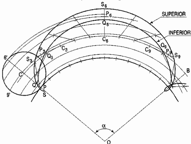
Epitrochoids
