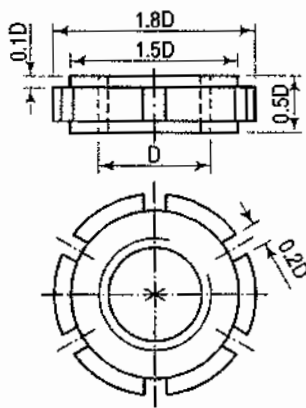
Ring nut
