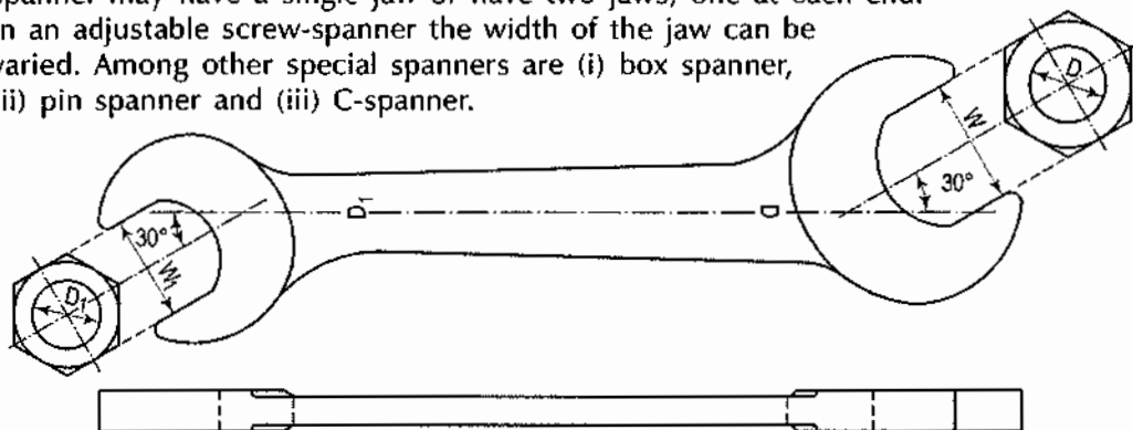
Spanner FIG. 24-72
