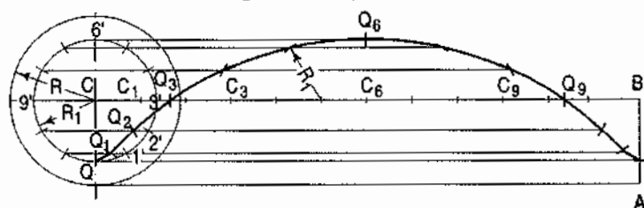
Inferior trochoid
