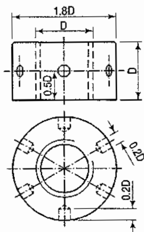
Capstan nut
