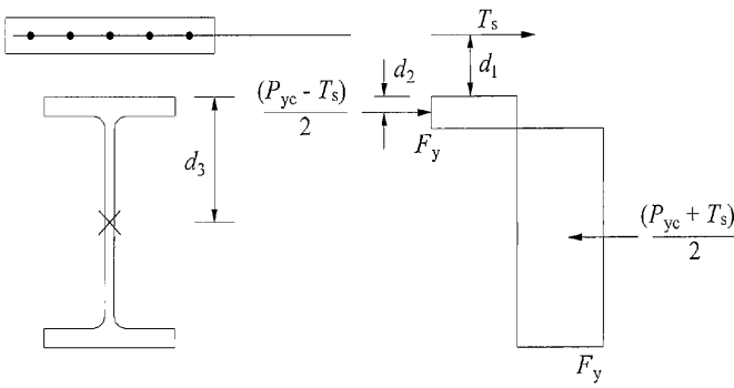
Şekil 12.3 – Kompozit kirişte negatif eğilme momenti için genel plastik gerilme yayılımı
