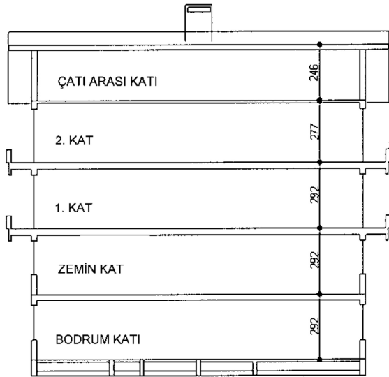
B – B KESİTİ
