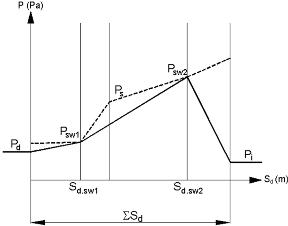
Şekil F.9 – Bir ara yüzde buharlaşma ve iki ara yüzde yoğuşmanın olduğu durum
