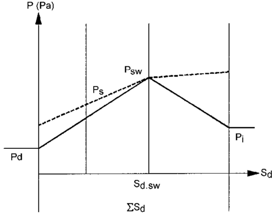
Şekil F.7 – Yapı bileşeninin bir ara yüzündeki buharlaşma
